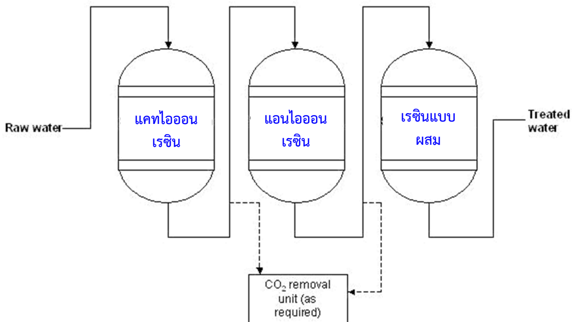
ภาพที่ 5-2 ระบบผลิตน้ำปราศจากไอออน ที่มีการเพิ่มขั้นตอนการใช้เรซินแบบผสม ติดตั้งหลังจากการกรองผ่านแคทไอออนเรซิน และแอนไอออนเรซิน เพื่อดักจับไอออนที่หลุดรอดมาจากขั้นตอนก่อนหน้า
