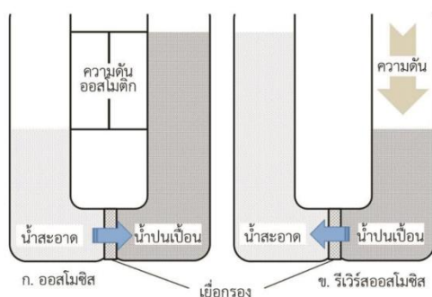
ภาพที่ 4-1 กระบวนการออสโมซิส และรีเวิร์สออสโมซิส
